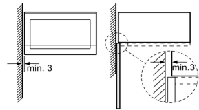
Rozměry v mm
